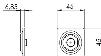
Adaptateur 45 anti-rotation 10 roulette pivotante
