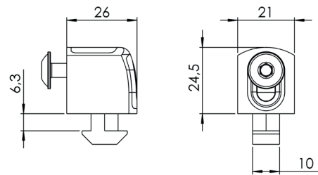
Panoblock 10 PA sécurité avec vis
