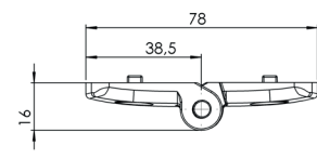
Charnière Al 40x40 E=45mm
