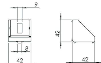
Kit équerre 8 x45x45x45 Al brut avec cache
