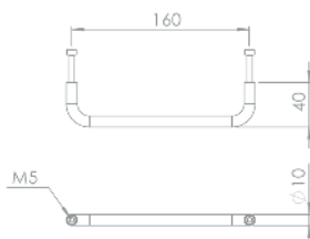
Kit poignée Al 160
