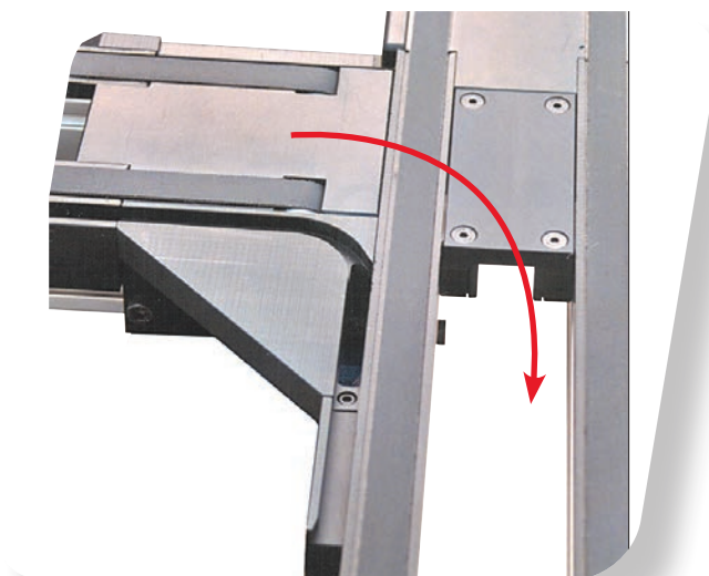
Cam 90° SD
