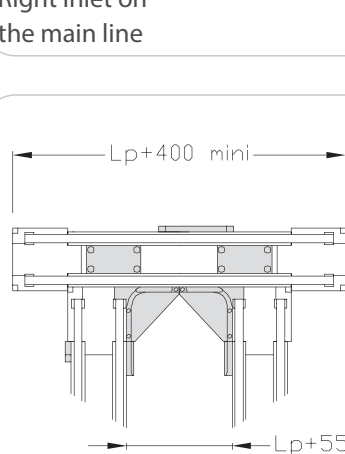
Cam ED
